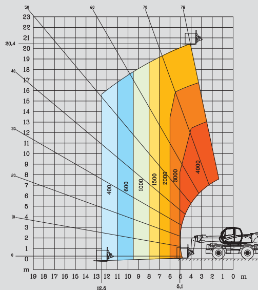
ROTATIE OP UITGESCHOVEN STEMPELS MET LIER 5 T
