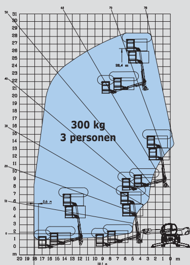
ROTATIE MET UITGESCHOVEN STEMPELS MET WERKKOOI AREAL JIB
