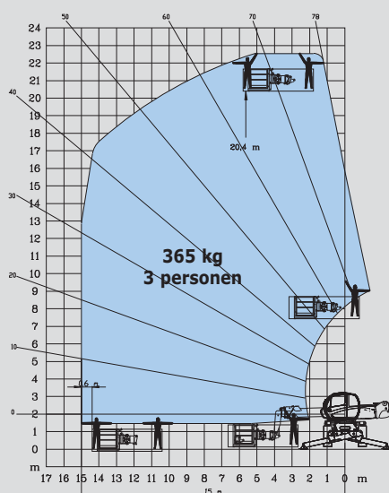
ROTATIE MET UITGESCHOVEN STEMPELS MET 3D-PLATFORM POSITIEVE WERKZONE
