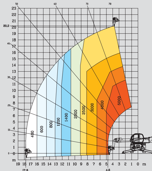
ROTATIE MET UITGESCHOVEN STEMPELS MET KRAANBALK P 1500
