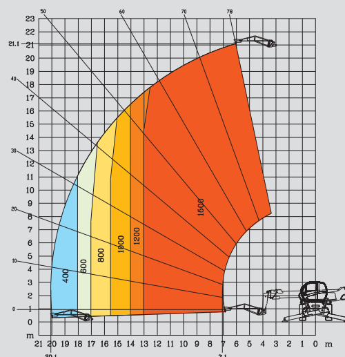
ROTATIE MET UITGESCHOVEN STEMPELS MET KRAANBALK P 1500
