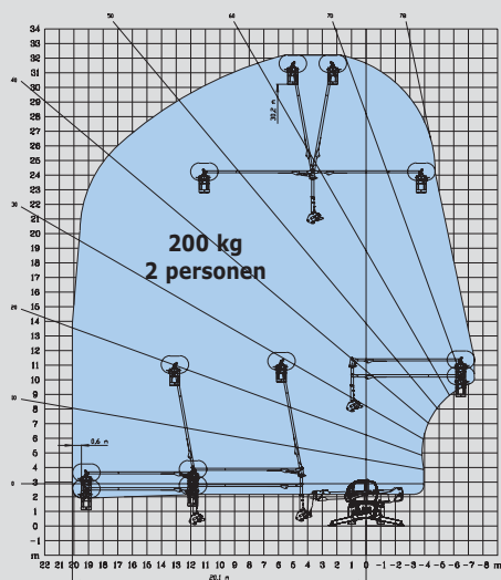
ROTATIE MET UITGESCHOVEN STEMPELS MET WERKKOOI AREAL JIB
