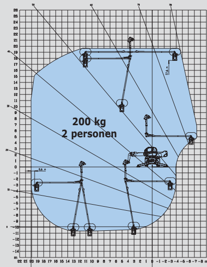
ROTATIE MET UITGESCHOVEN STEMPELS MET KRAANBALK
