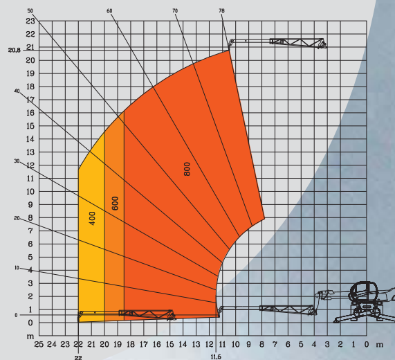
ROTATIE MET UITGESCHOVEN STEMPELS MET KRAANBALK
