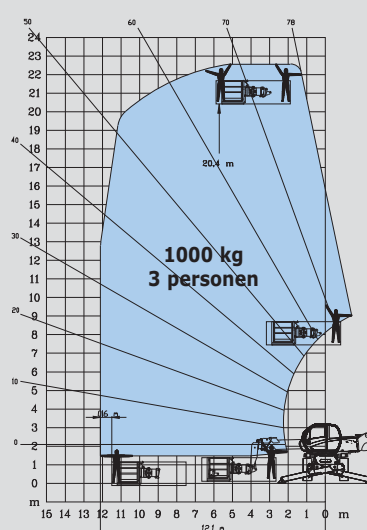
ROTATIE MET UITGESCHOVEN STEMPELS MET WERKKOOI 1000 KG 2,25/4 M
