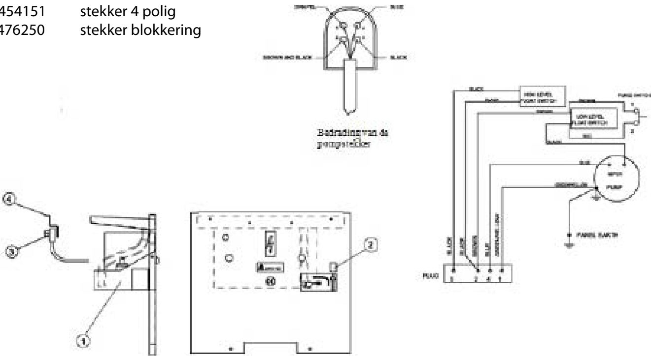
Elektrisch schema condenswaterpompkit
