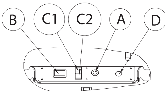
Fig. 39 Bedieningspaneel
