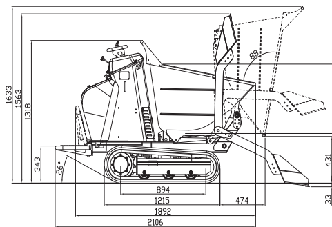
Fig. 10 Technische gegevens zelfladende versie
