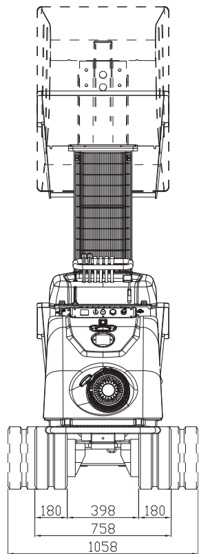
Fig. 18 Technische gegevens versie extra hooglosser
