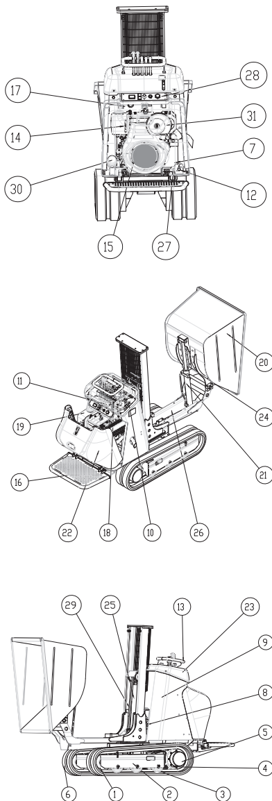
Fig. 22 Begrippen componenten machine
