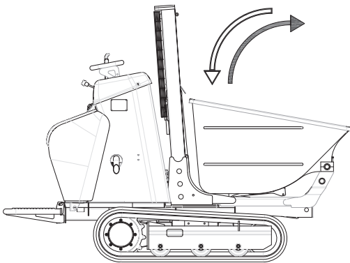
Fig. 43 Vast onderstel
