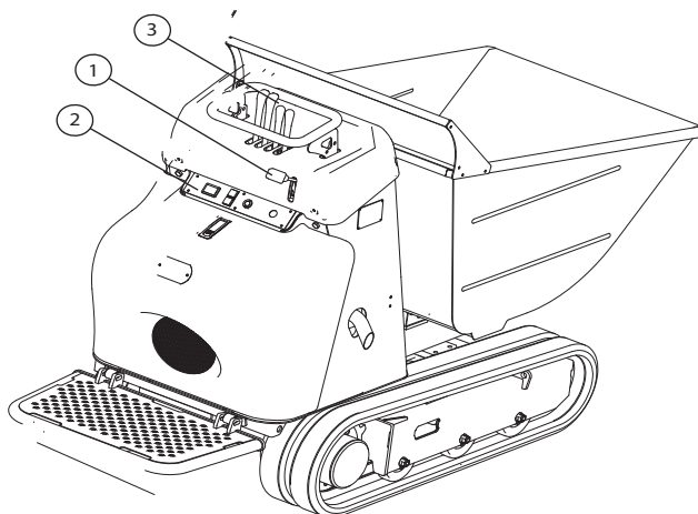
Fig. 36 Positie van de bedieningsorganen Dieselversie
