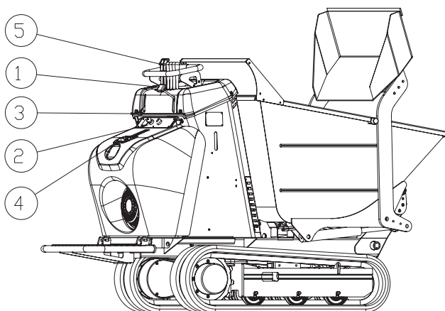
Fig. 35 Positie van de bedieningsorganen benzineversie
