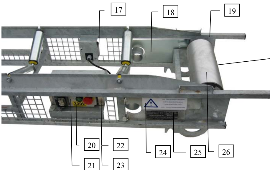
MOTORZIJDE TRANSPORTBAND
